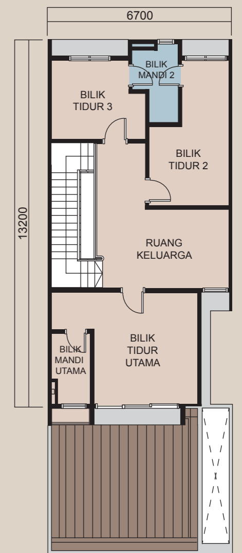
PELAN LANTAI TINGKAT SATU
